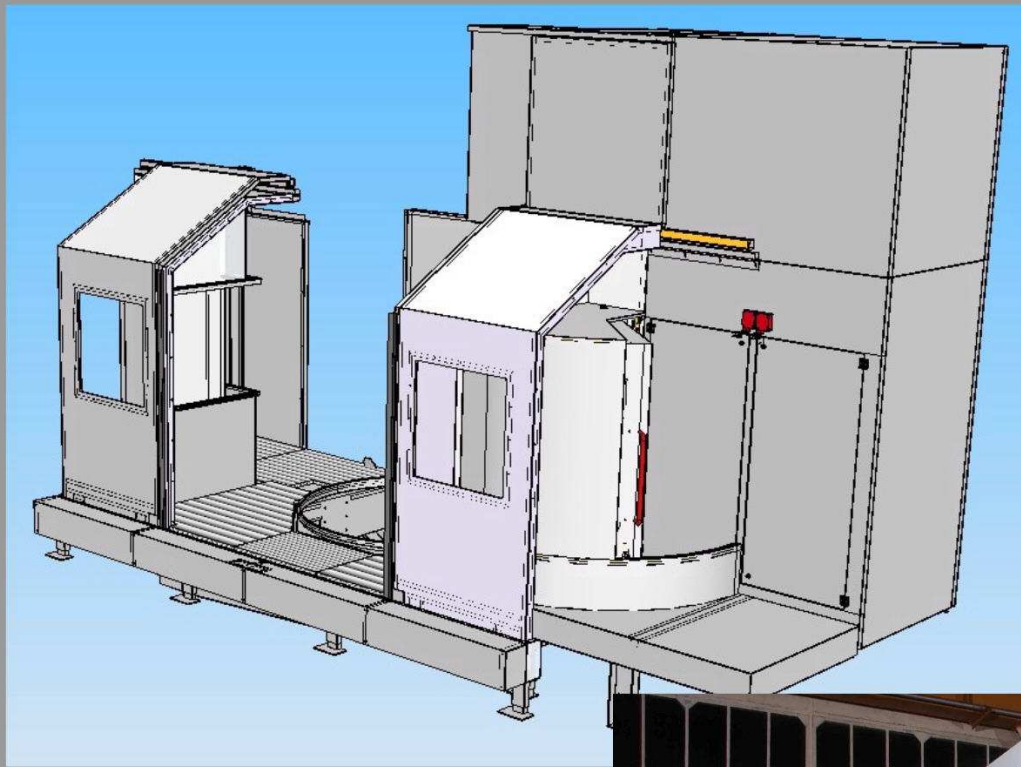
Rectifieuse verticale Diam 2000 2 portes chargement meule manuelle et automatique
